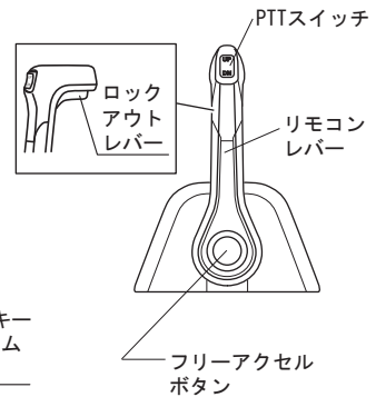
トップマウントタイプ リモートコントロールボックス仕様
